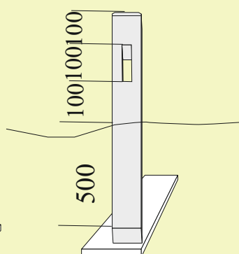
Poteau à mortaise débouchante
