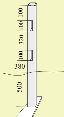
Poteau à mortaises débouchantes
